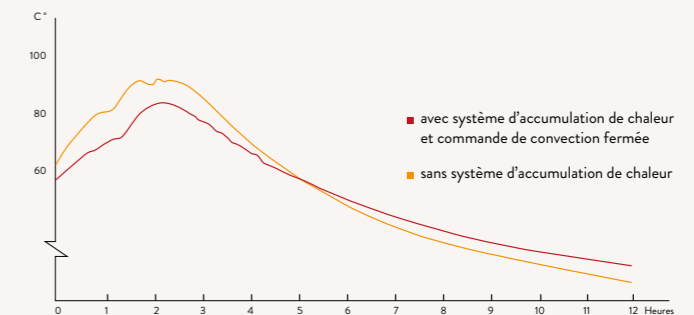
Ce graphique représente la déperdition de chaleur après le dernier chargement.
